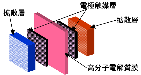
MEA模式図
