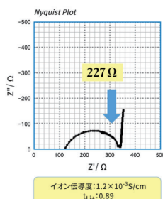
ゲルポリマーイオン伝導度・輸率
